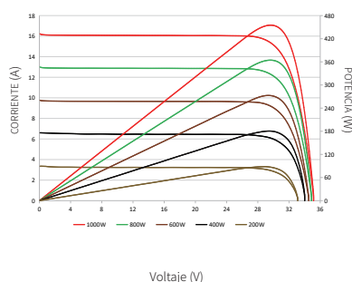
Curvas de corriente-voltaje y potencia-voltaje (445W)
